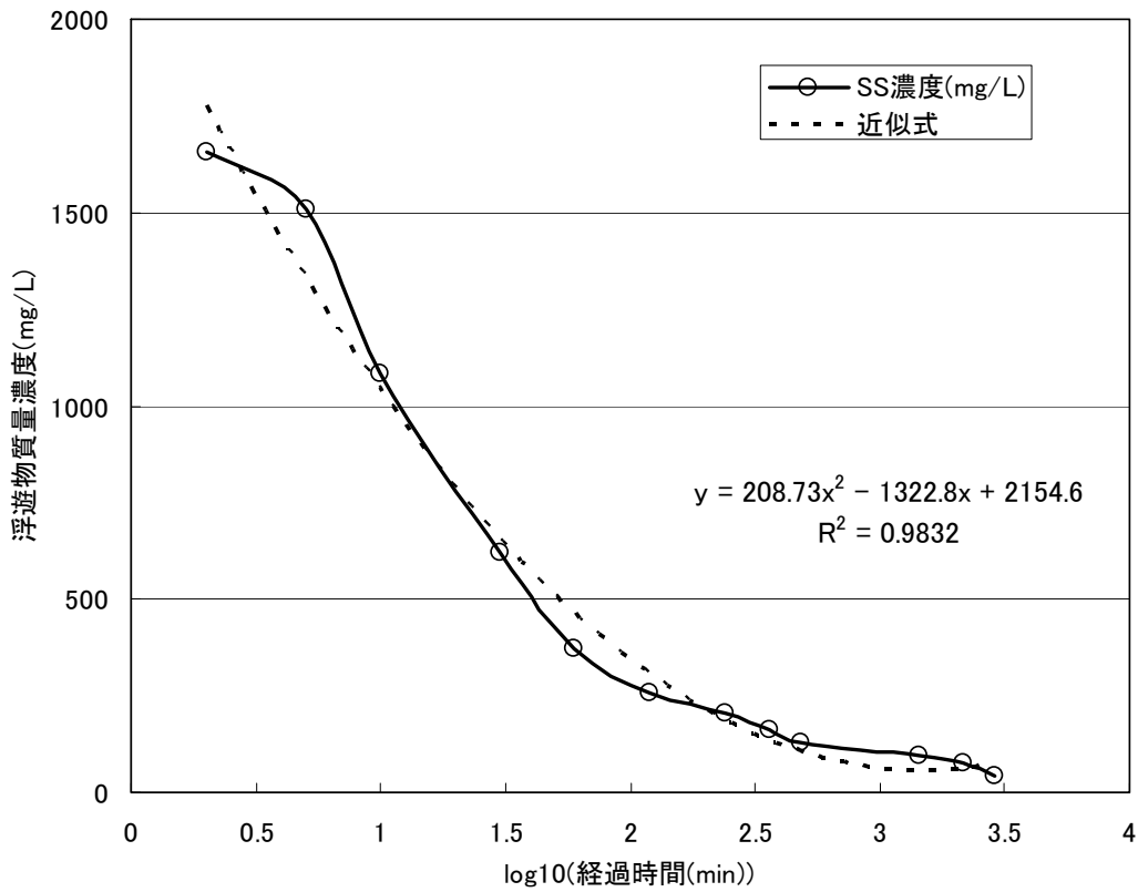
図 8.6.2-2 沈降試験結果から算出した近似式
