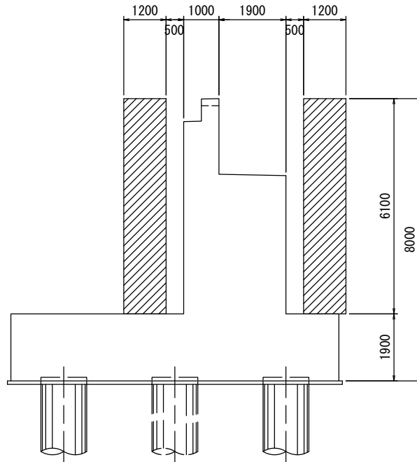
橋台躯体工足場参考図
