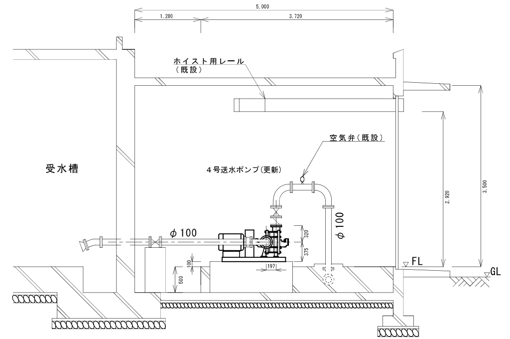
B-B'断面図
