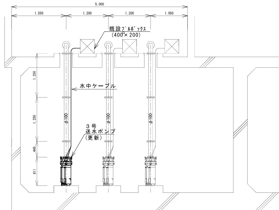
A-A'断面図
