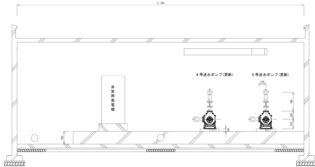
A-A'断面図
