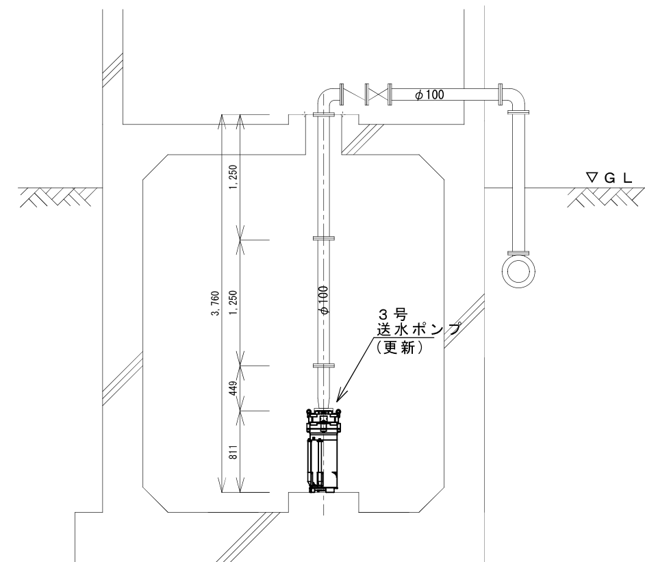
B-B'断面図
