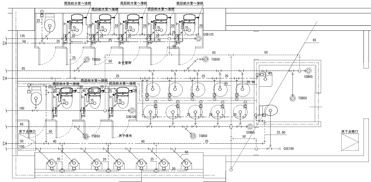
1階①平面詳細図（改修後） S=1/40
