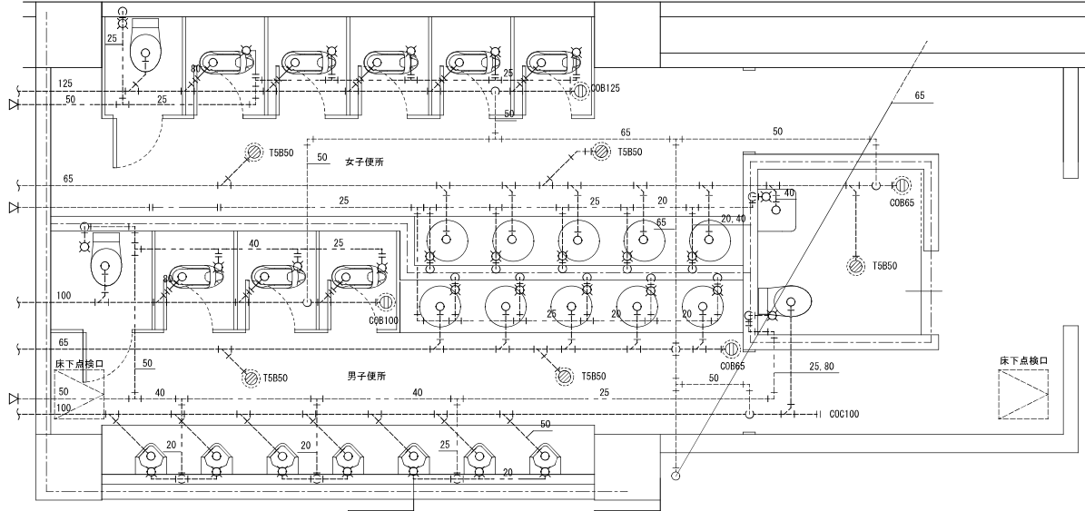
1階①平面詳細図（改修前） S=1/40
