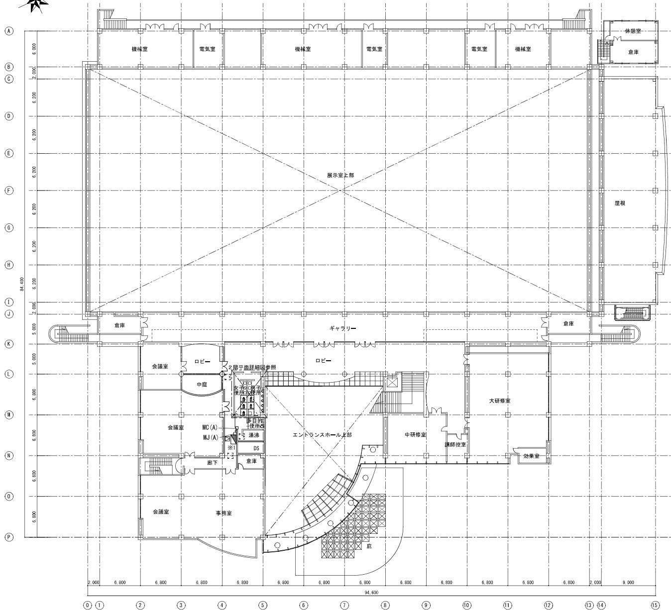
2階平面図 1/300
