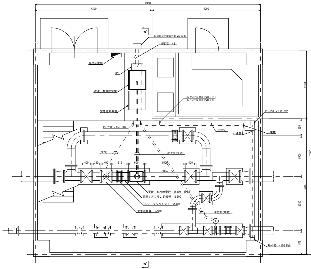
平面図 S=1:30
