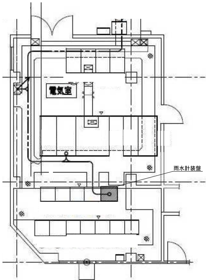
電気室平面図
