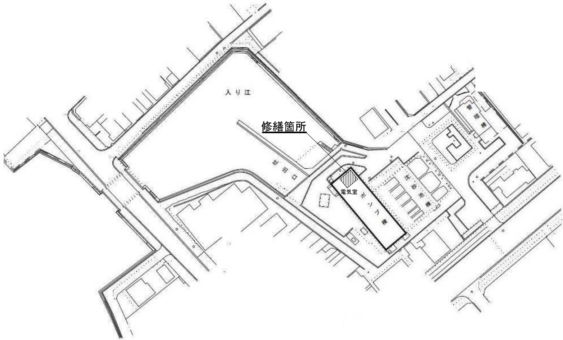
極楽橋ポンプ場全体配置図
