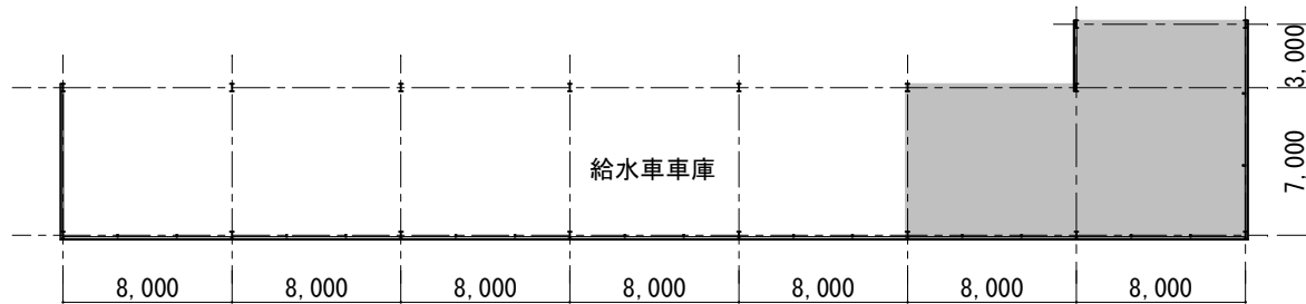
給水車車庫 平面図
