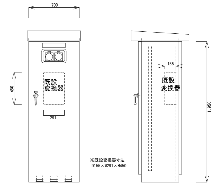
配水池盤 1/30
