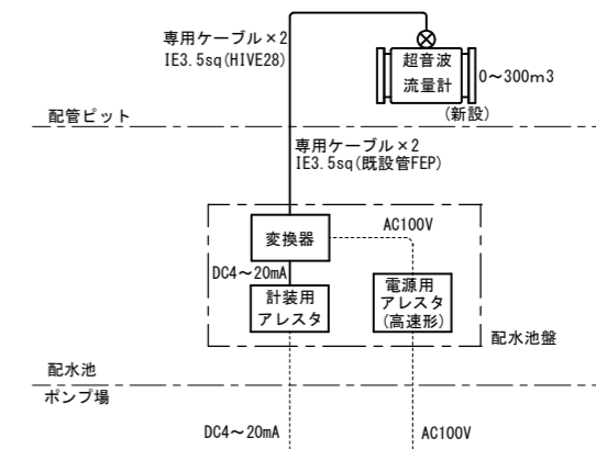
配水池盤 1/30
