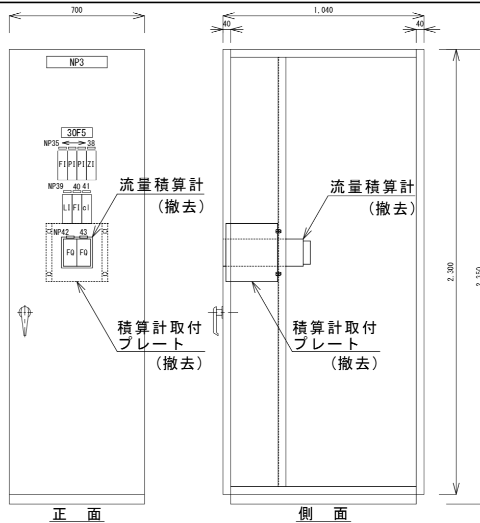
計装盤 (更新前)
