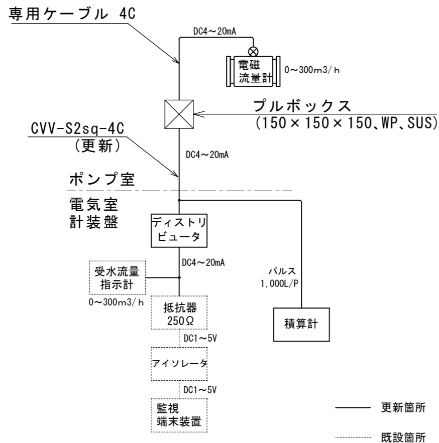
受水流量計系統図
