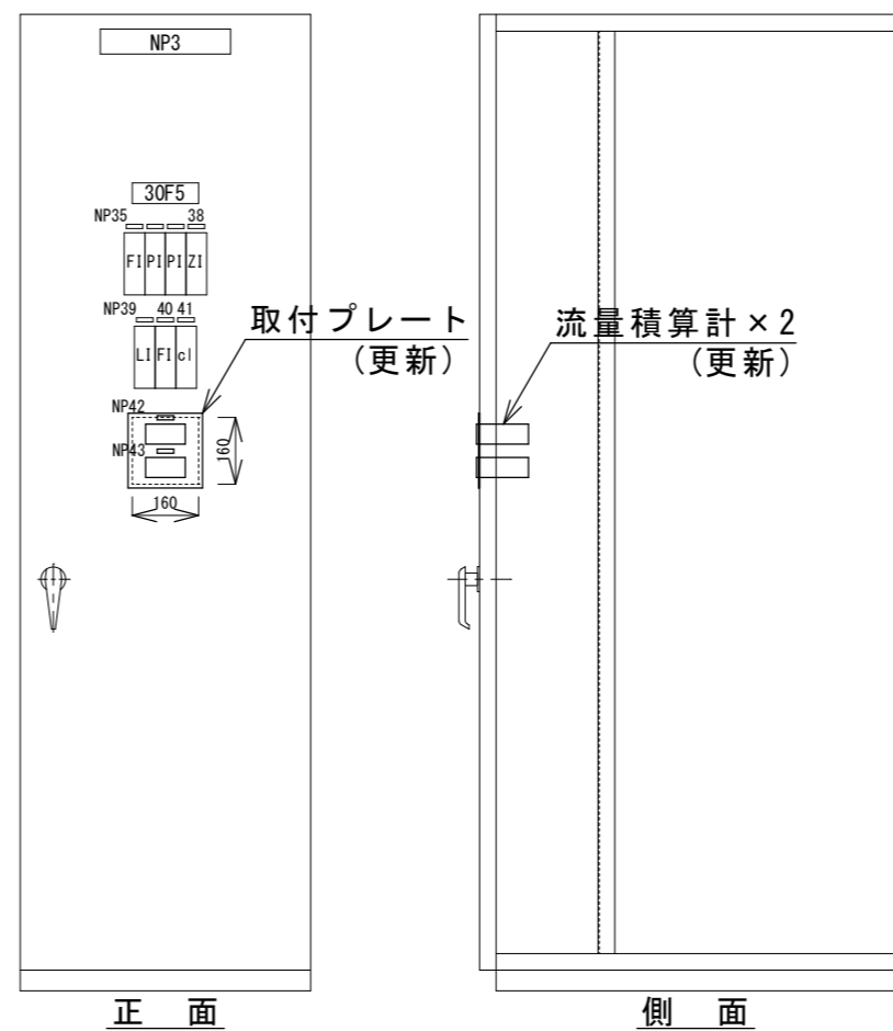
計装盤 (更新後)
