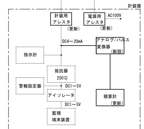
配水流量計系統図
