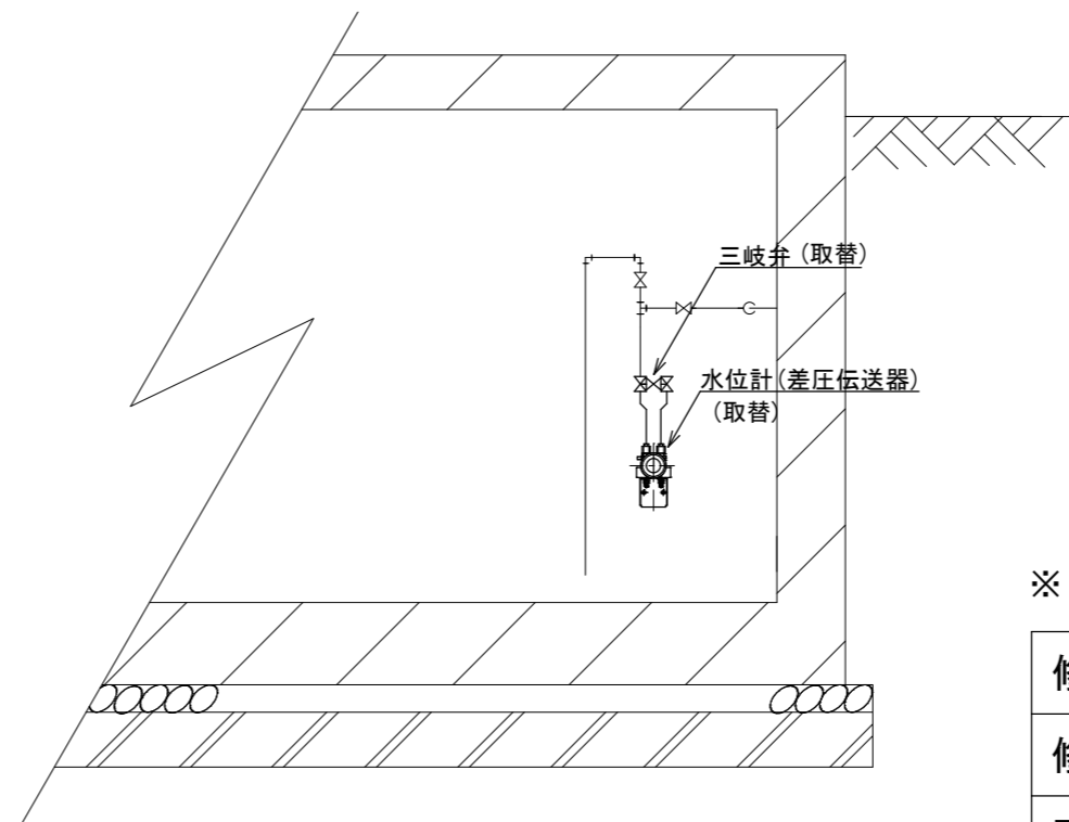
A-A' 矢視 1/30
