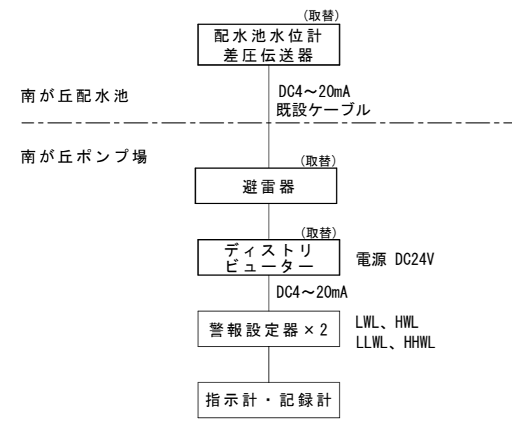
系統図
