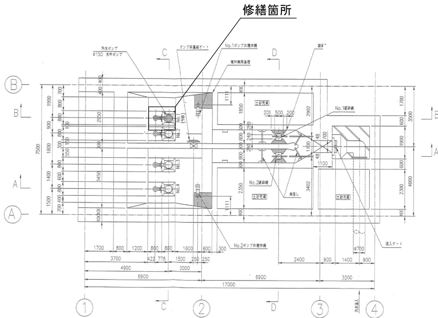
水路平面図
