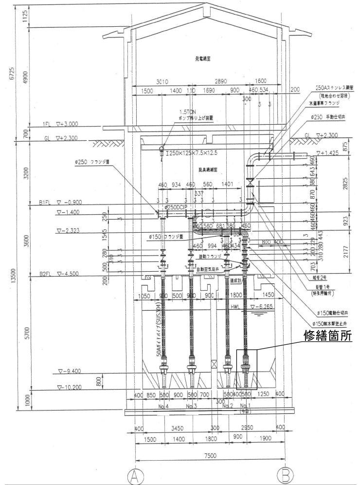
C-C断面図
