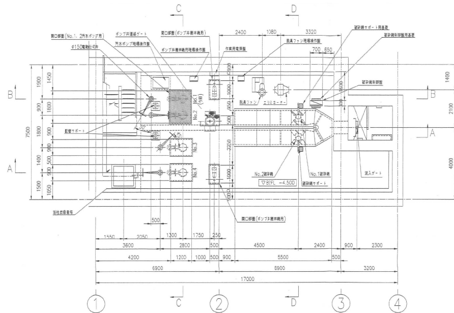
B2F平面図
