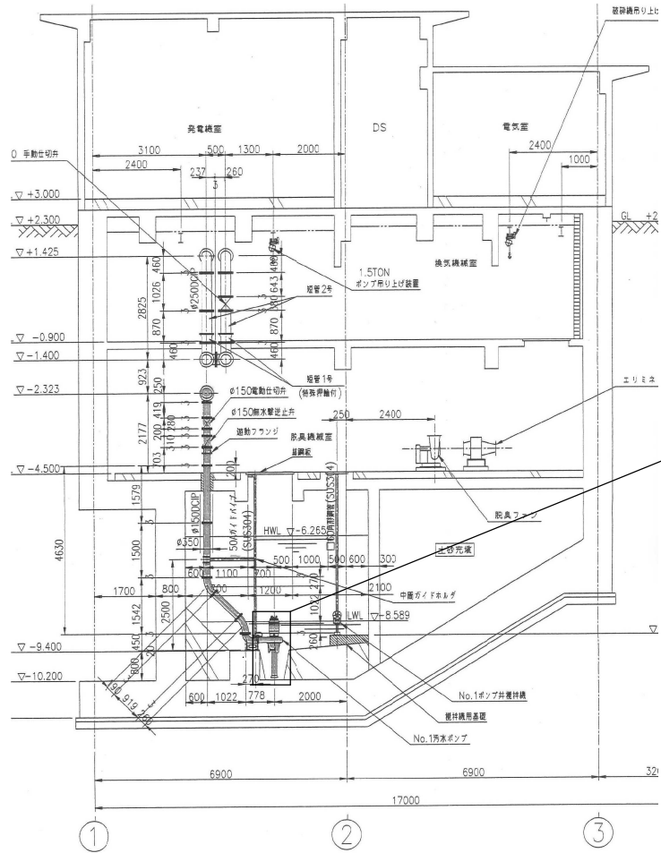
B-B断面図
