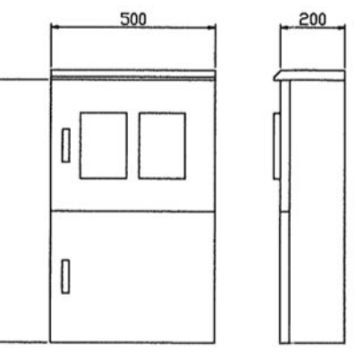
引込開閉器箱参考外観図 S=1/10
