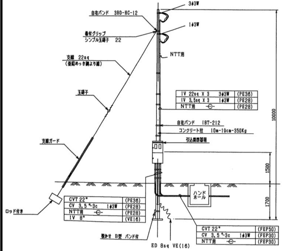
引込柱図 S=1/50
