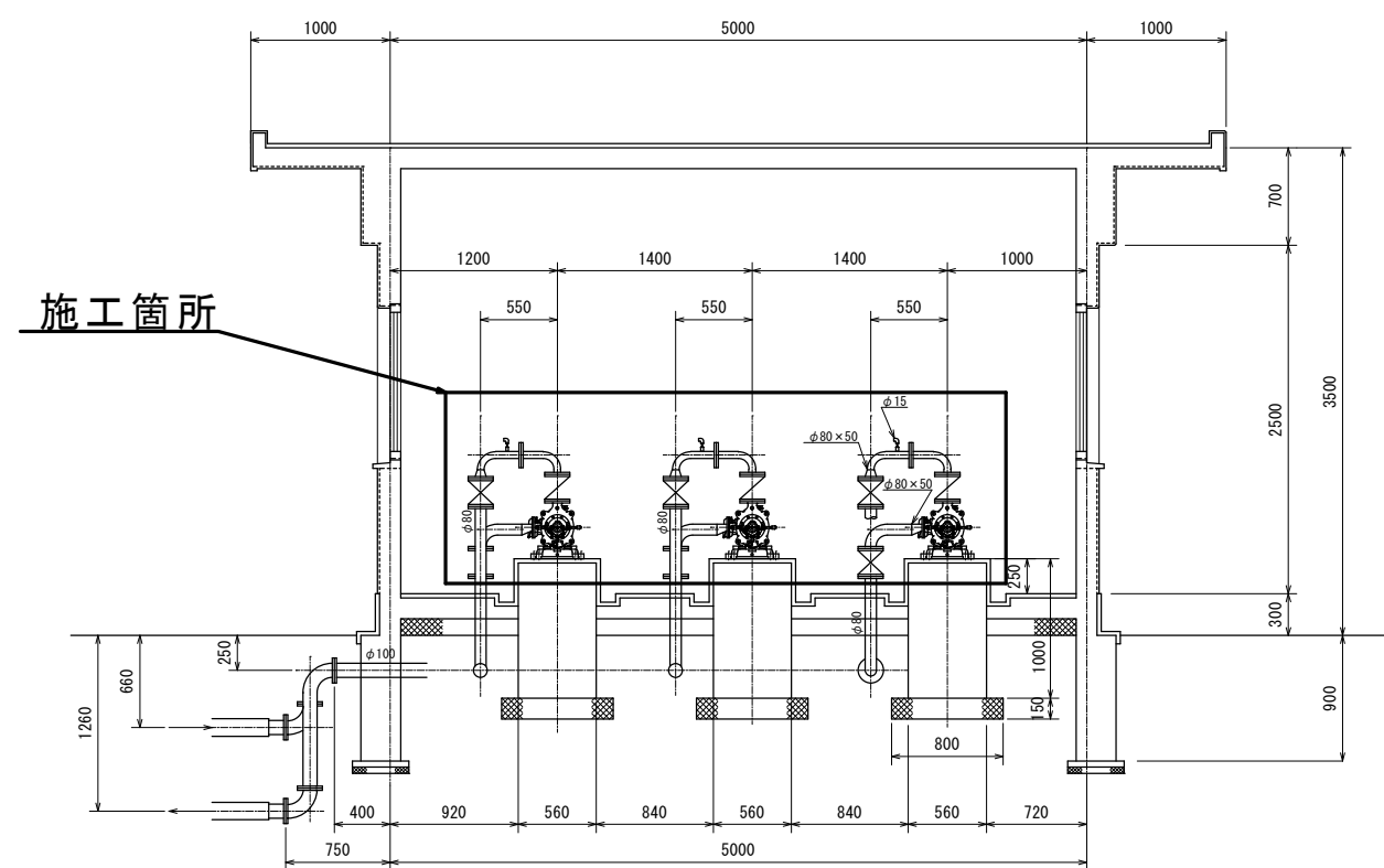
B-B 断面図
