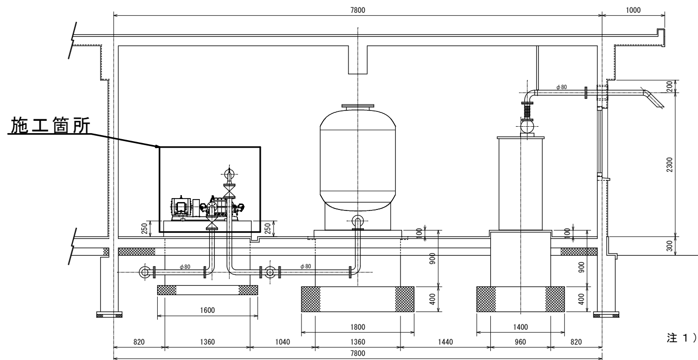
A-A 断面図
