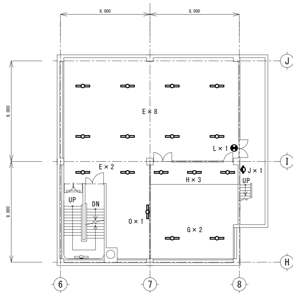
地階平面図 S=1:200
