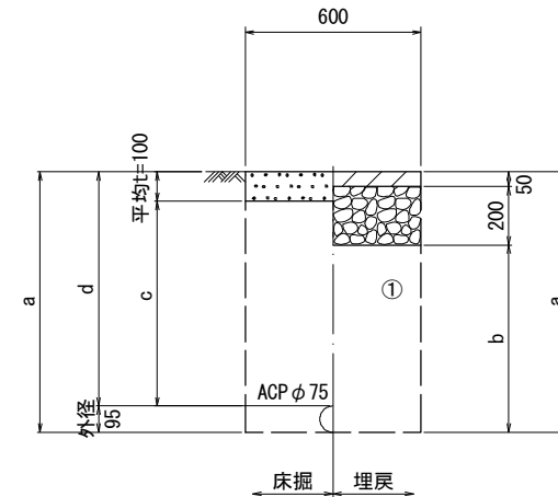
既設管撤去
