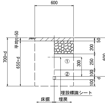
給水管
