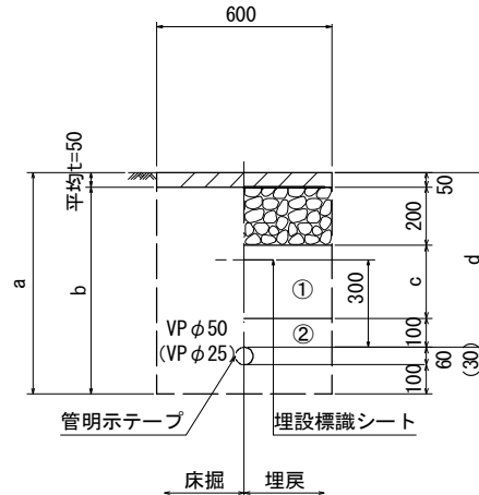
泥吐管
