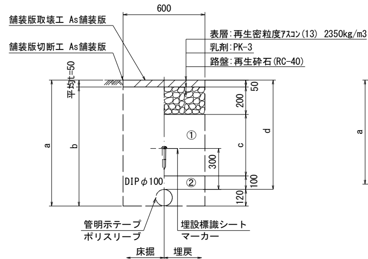
GXφ100
